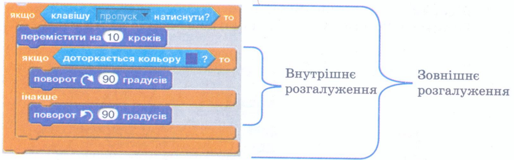
Мал. 3.30. Приклад вкладеного розгалуження в Scratch
