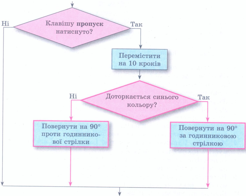
Мал. 3.31. Блок-схема фрагмента з вкладеними розгалуженнями в Scratch
